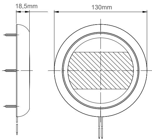
Afm. ø130 x 18,5mm
