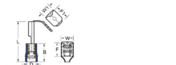
GEISOLEERDE VLAKSTEKERHULS MET EXTRA TAB PIGGY BACK - VORISOLIÈRT DOPPEL FASTON
